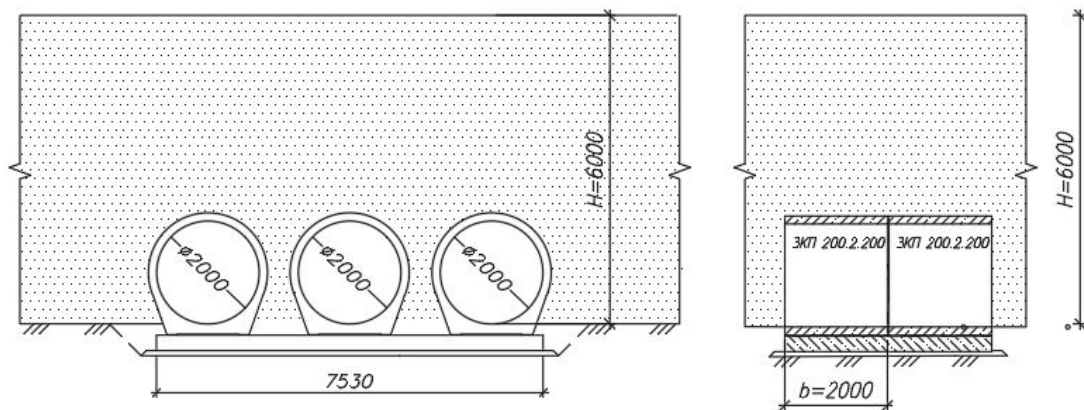
1 – Расчетная схема
